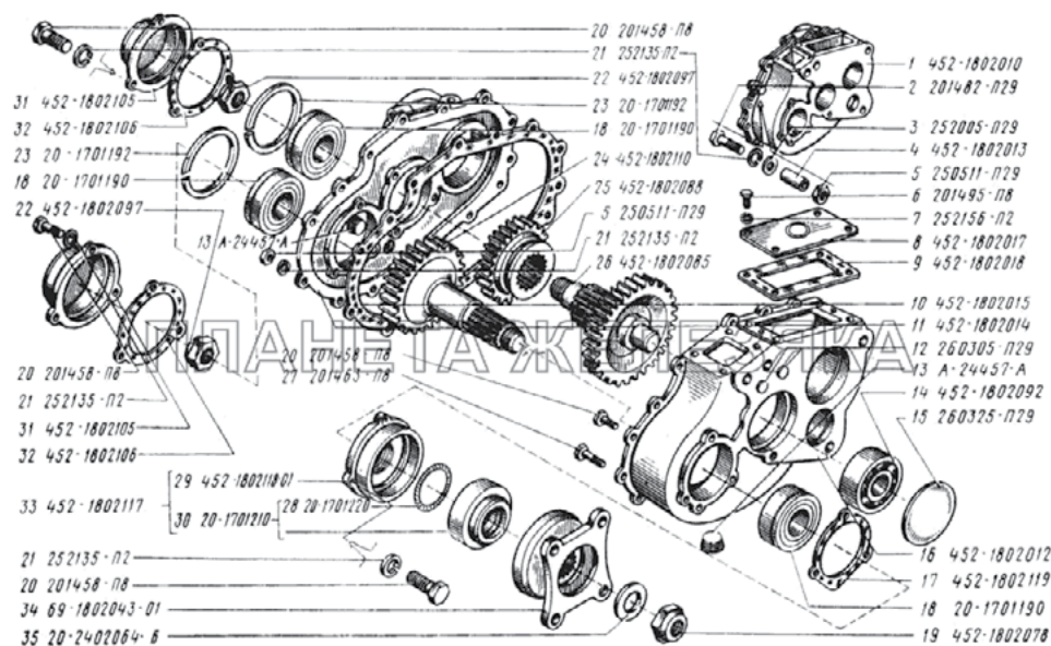
Рис. 52. Коробка раздаточная (1802)/1
