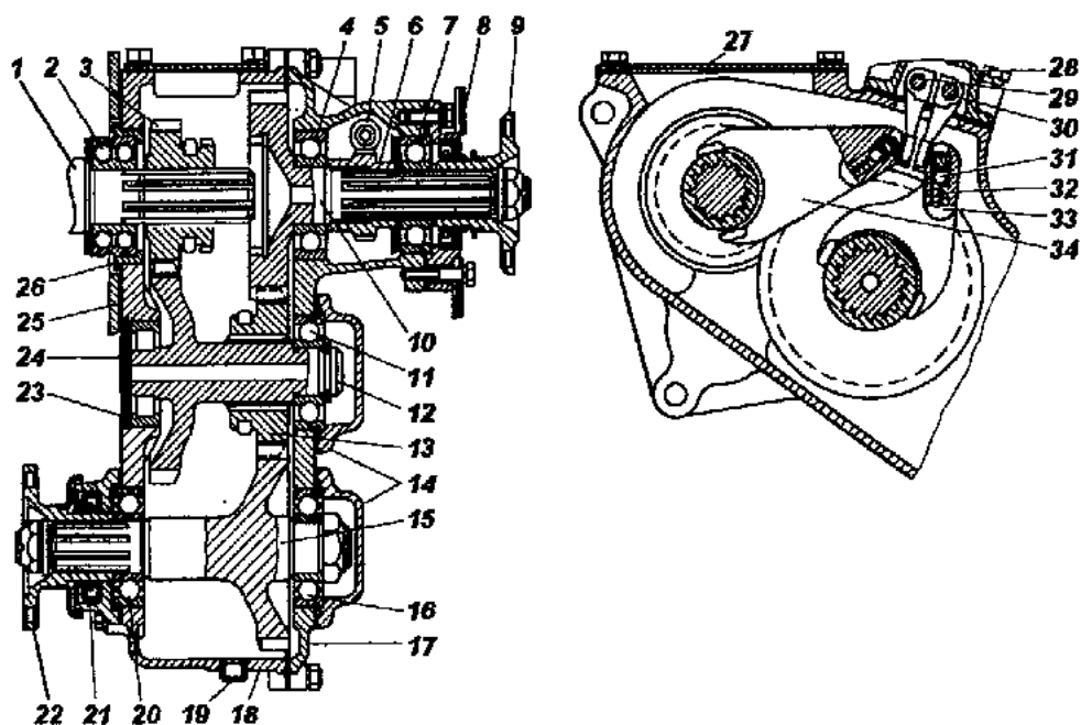
Рис. 52. Коробка раздаточная (1802)/1
