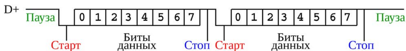
Рис. 1. Последовательность интерфейса UART
