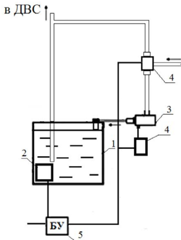
Рис. 1. Устройство для безразборной очистки деталей двигателя внутреннего сгорания от нагара 1 — бак; 2 — деспиргатор; 3 — смеситель; 4 — управляемый клапан; 5 — блок управления
