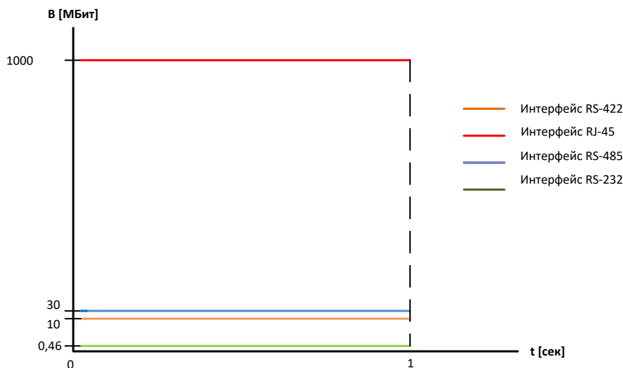
Рис. 4. График скоростей передачи информации интерфейсов: RS-232, RS-422, RS-485 и RJ-45
