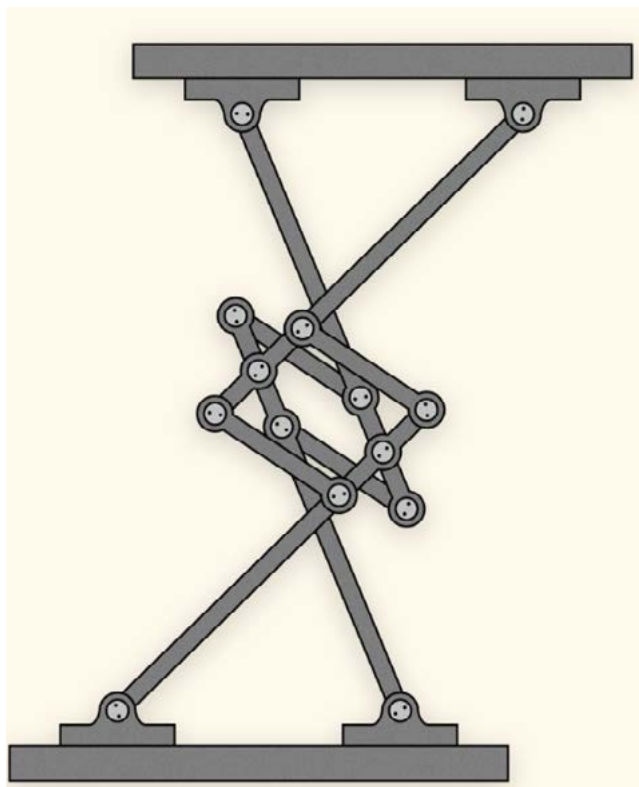
Рис. 2. Схематическое изображение Табурета Чебышева [3]
