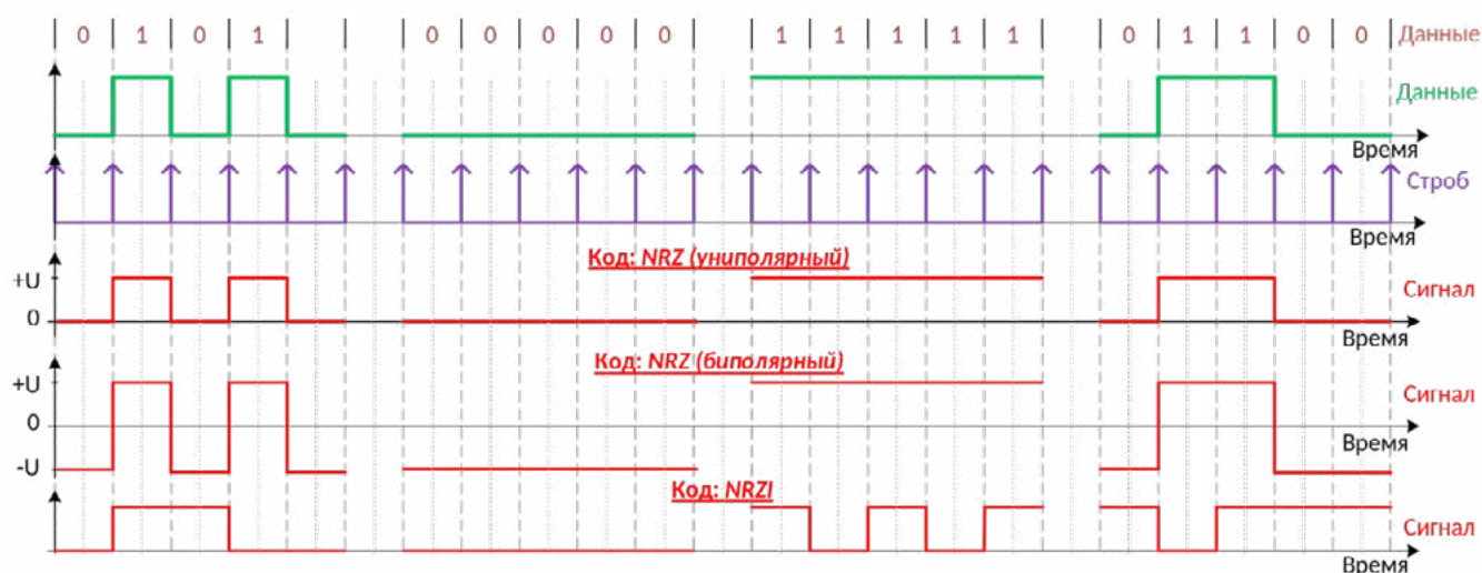
Рис. 2. Код NRZ
