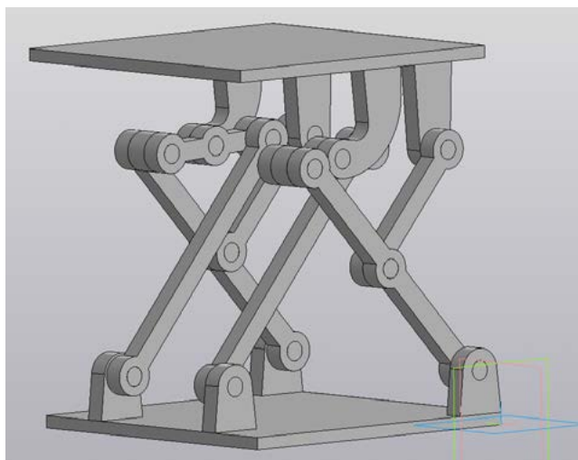
Рис. 3. 3D модель Табурета Чебышева
