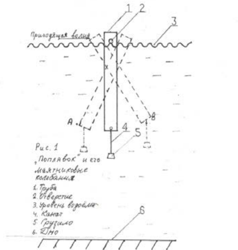
Рис. 1. «Поплавок» и его маятниковые колебания.
